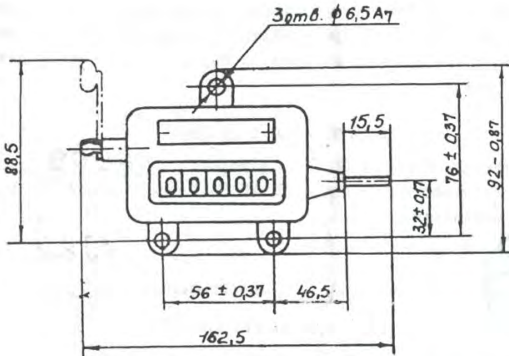
Габаритные, установочные и присоединительные размеры счетчика
